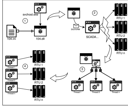
(d) IEC-104 payload
